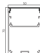
PR-LS-SL-5070 Универсальный 3000mm ● Серый ● Не анод
