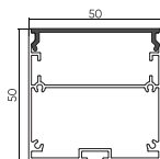
PR-LS-SL-5050 Универсальный 3000mm ● Серый ● Не анод
