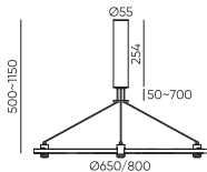
Трек подвесной круг ECLIPSE-MG-TRACK-RN Размеры: 500(1150)* \varnothing 650мм/800мм
