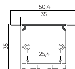
PR-LE-5035 Встраиваемый 3000mm ○ Белый ● Серый
