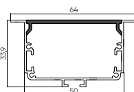
PR-LE-6434 Встраиваемый 3000mm ○ Белый ● Серый ● Не анод
