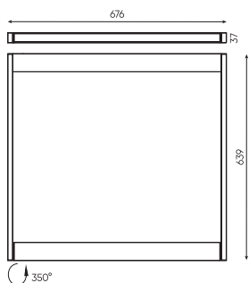
SATURN-SQS Накладной монтаж 24W | 1860Lm | 36°
